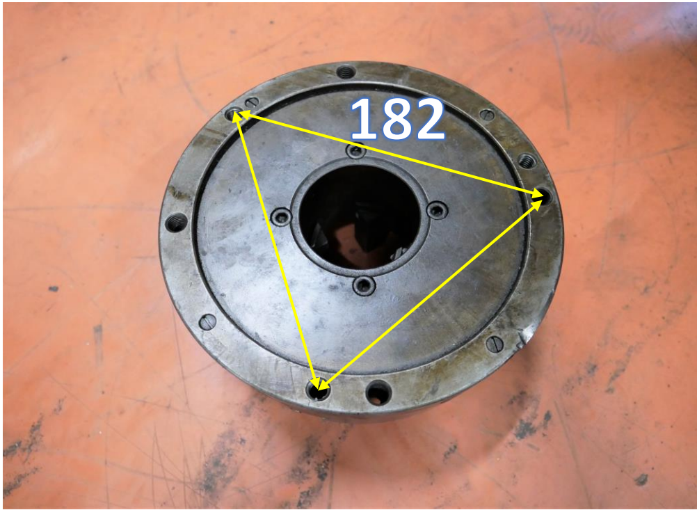
※裏から取付ける時、182ピッチ(3つ穴)
