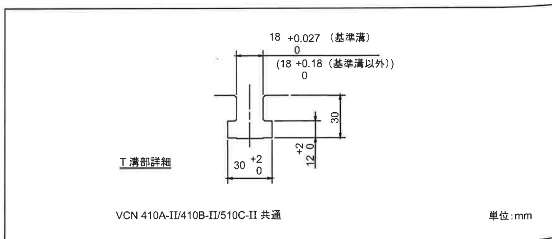
Fig. 1-7 T 溝形状
