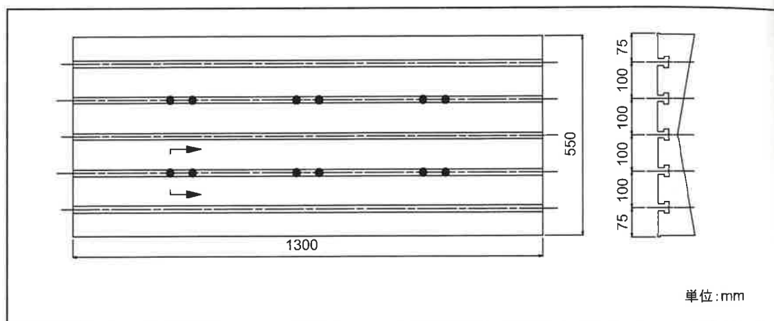
Fig. 1-6 テーブル寸法図 (VCN 510C-II)
