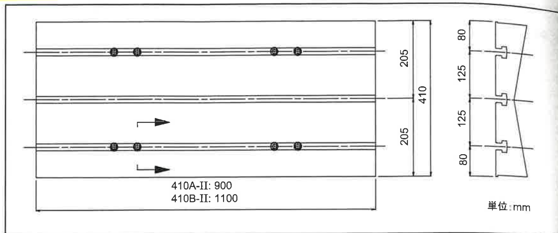
Fig. 1-5 テーブル寸法図 (VCN 410A-II/410B-II)
