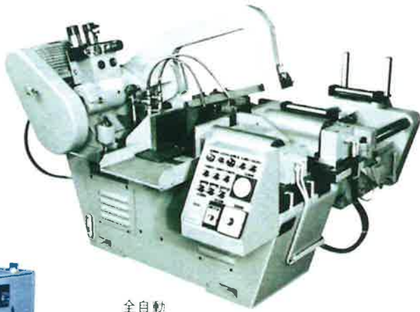
全自動 C-202AW ●200mm ■200×200mm (幅×高さ)
